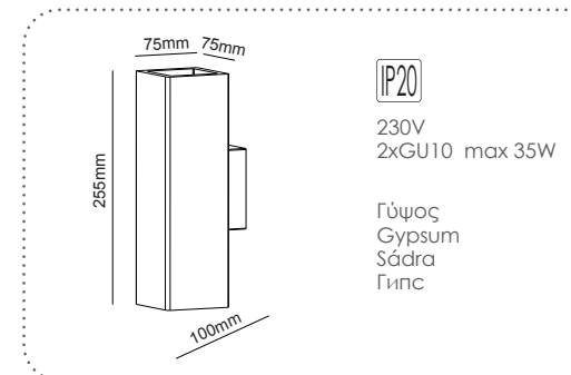
Επίτοιχο φωτιστικό Wall luminaire ILE
