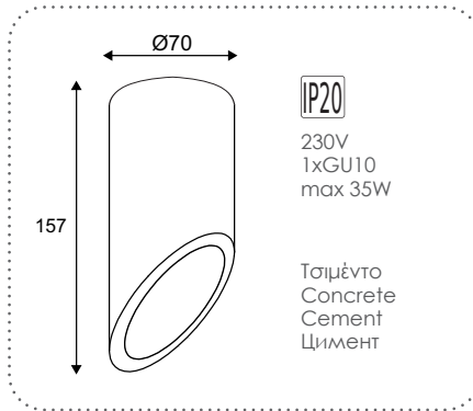
MK151S16G Φυσικό / Natural Přirodní / Естествен
